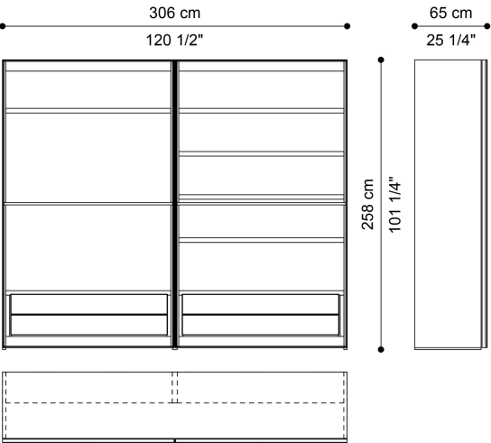
L 306 D 65 H 258 CM
